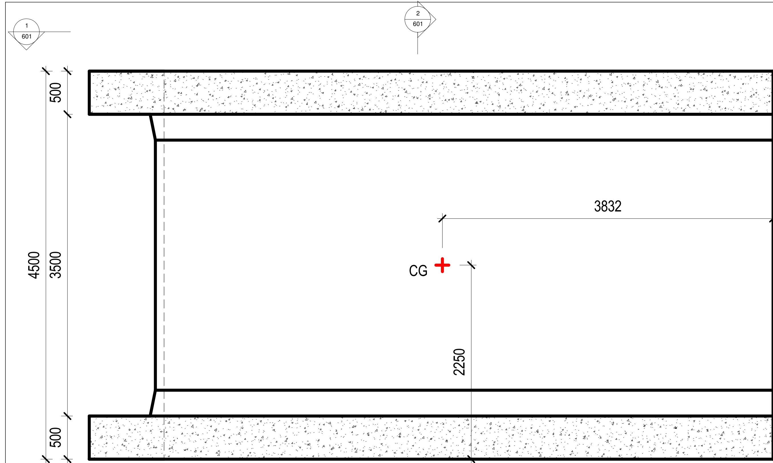
3 DETAIL SECTION B 1 : 25
