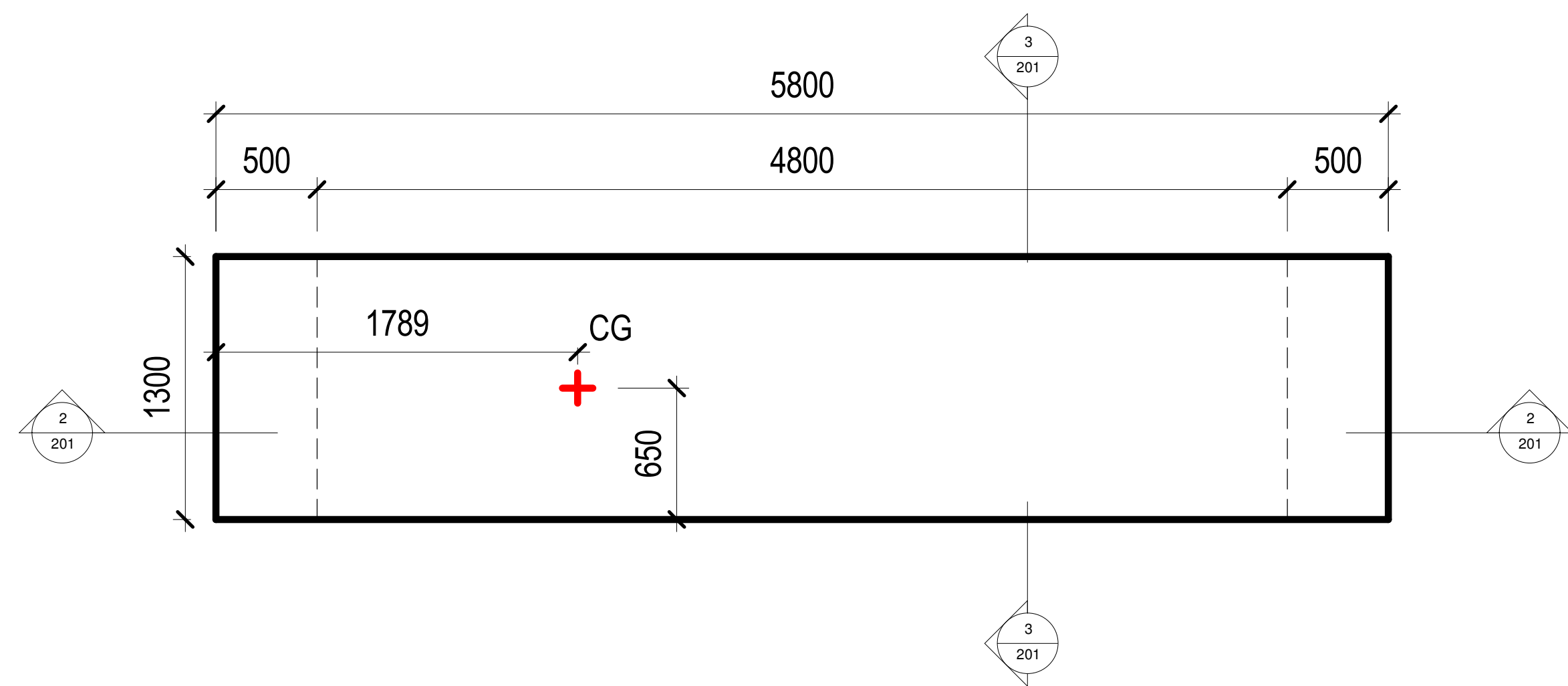
1 PLAN 1:25
