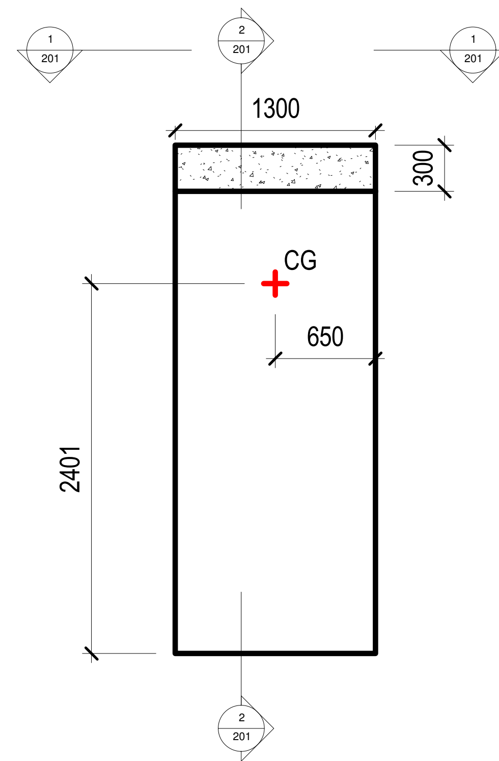
3 DETAIL SECTION B 1 : 25
