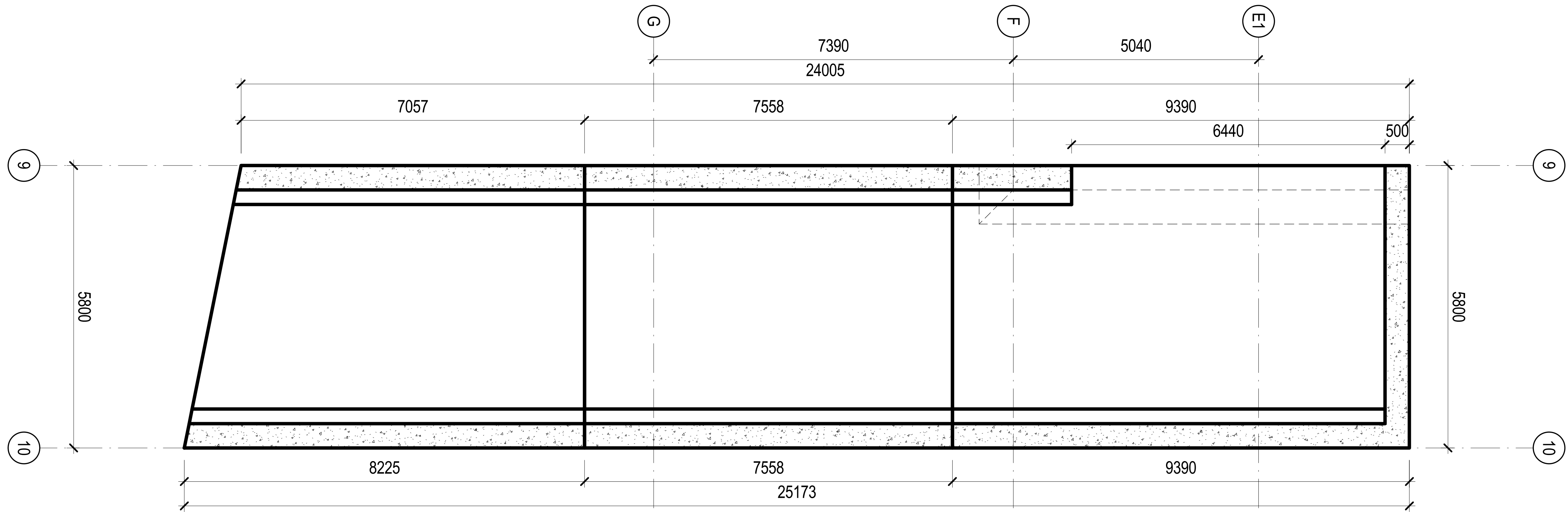
2 1 : 50 PLAN-CELL 9 -1.3
