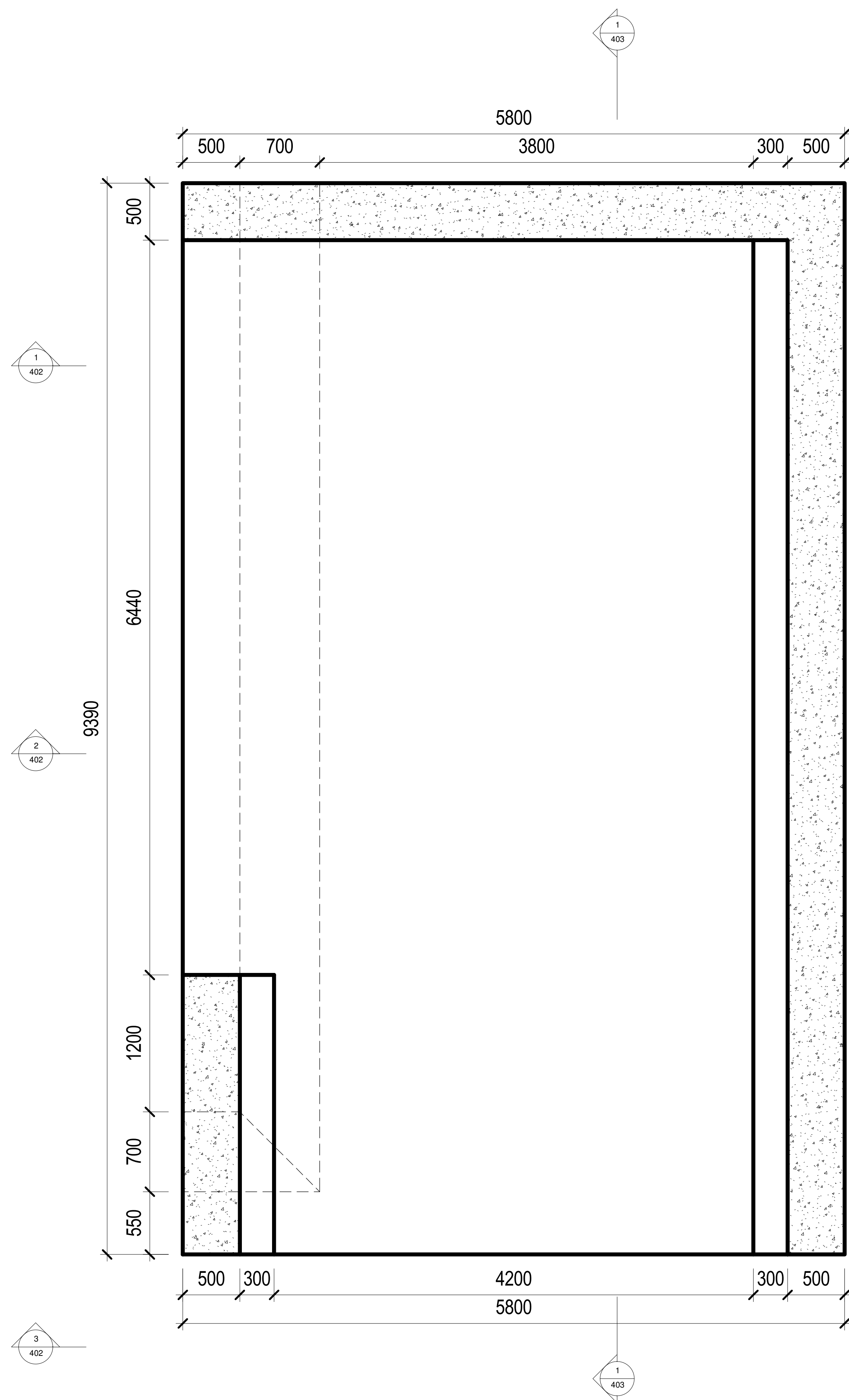
2 PLAN SECTION 1:25
