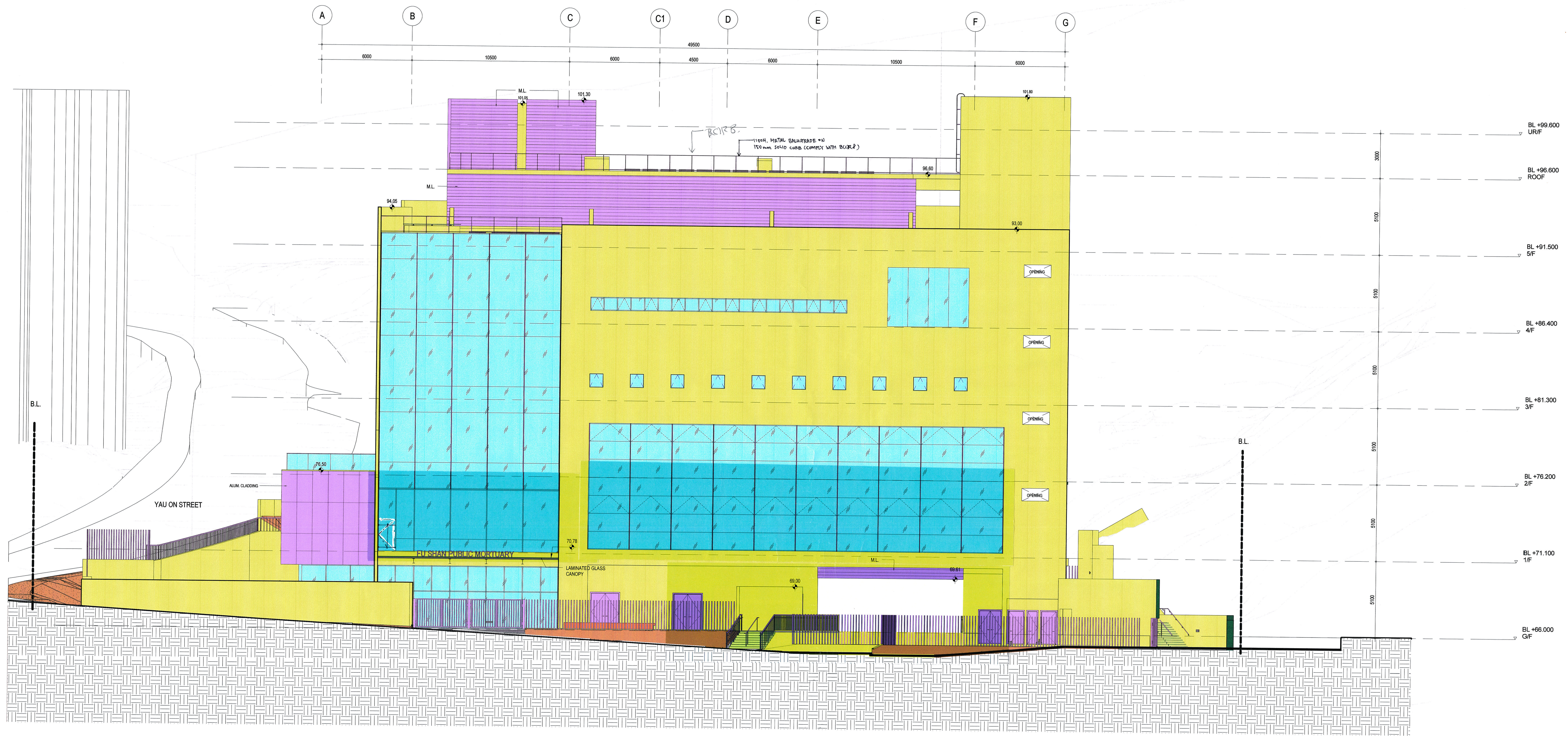
2 ELEVATION 1:100
