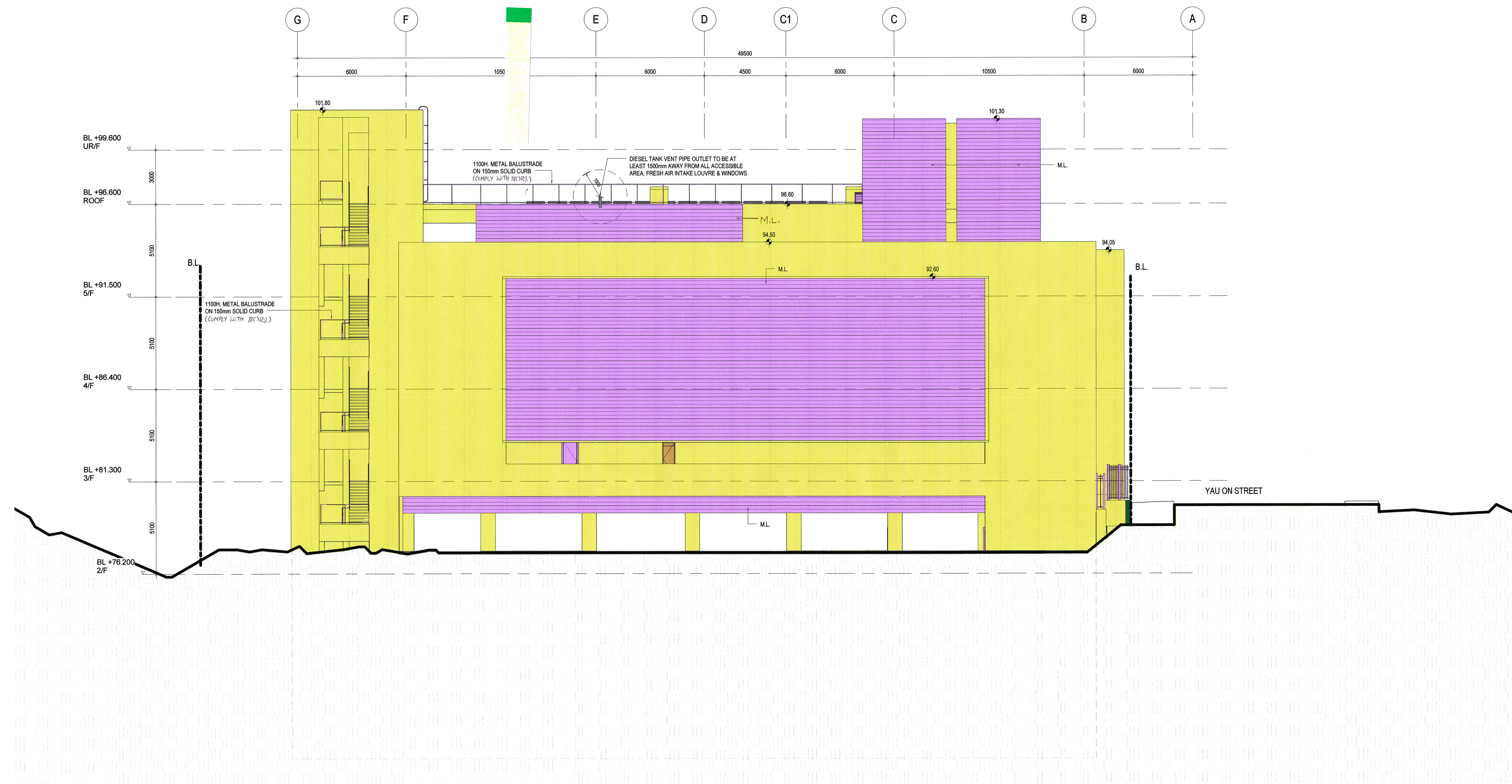
4 ELEVATION 1:100
