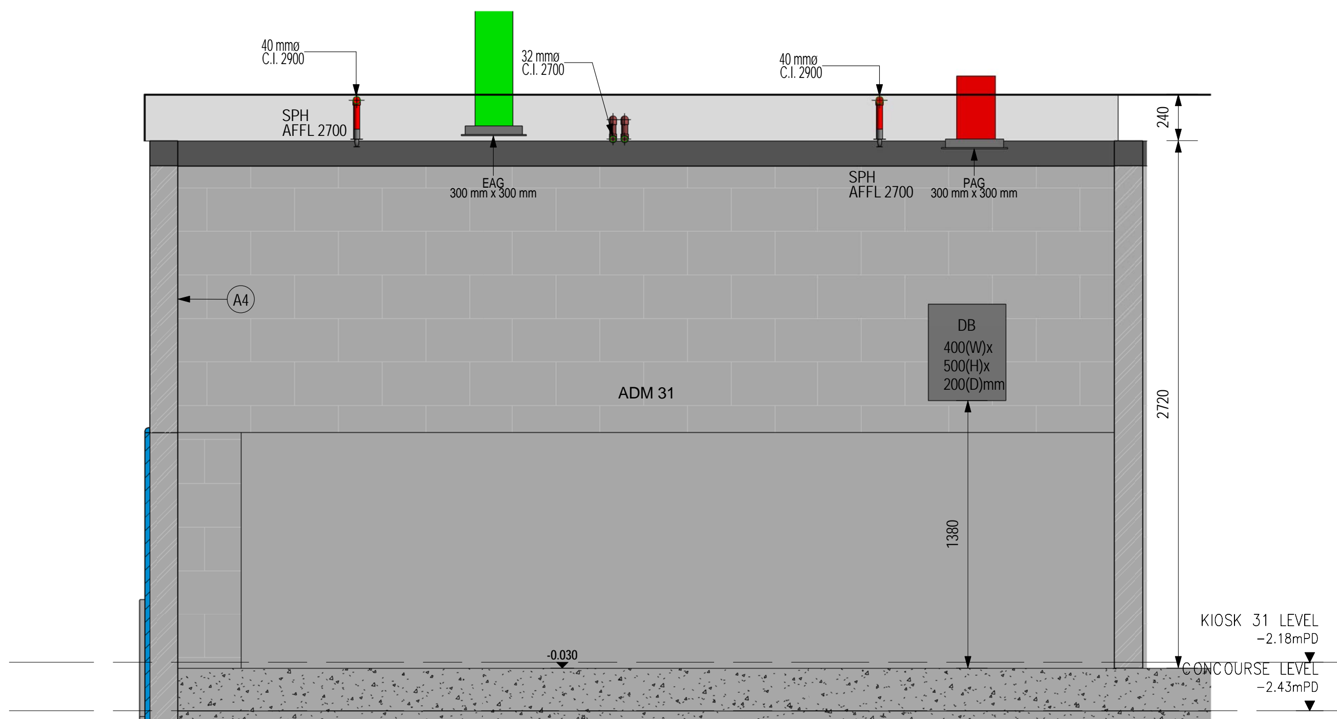
3 ELEVATION 3 1 : 20
