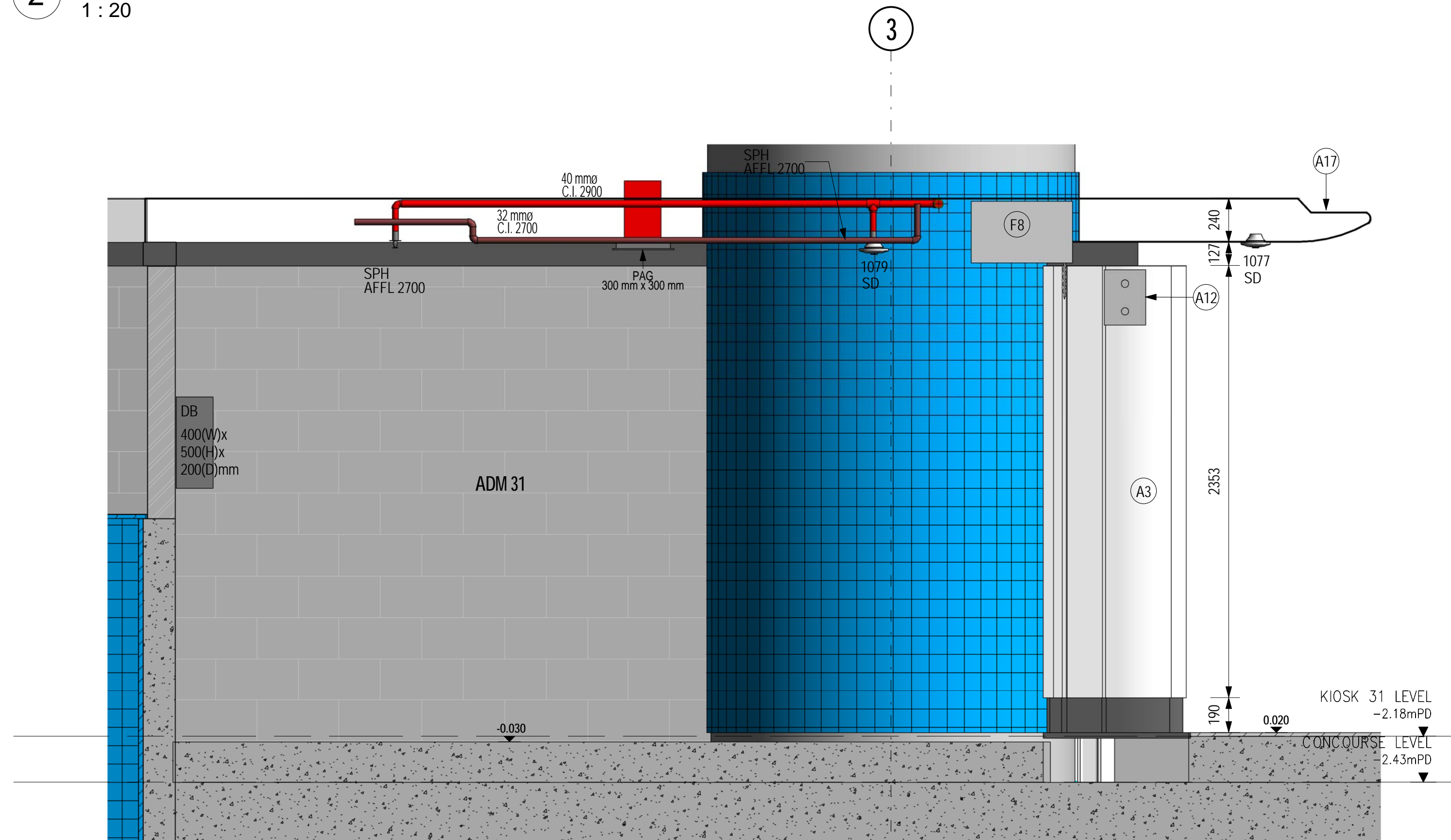
4 ELEVATION 4 1 : 20
