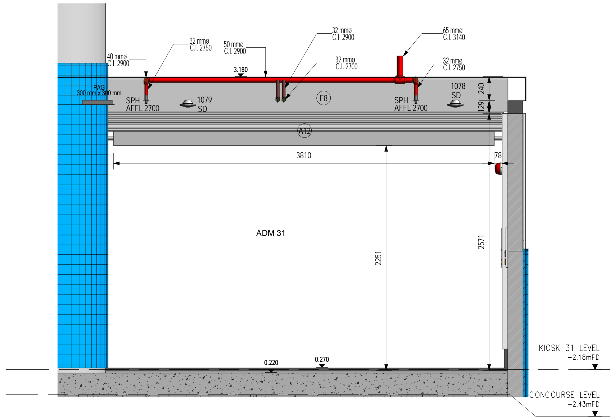
1 ELEVATION 1 1 : 20
