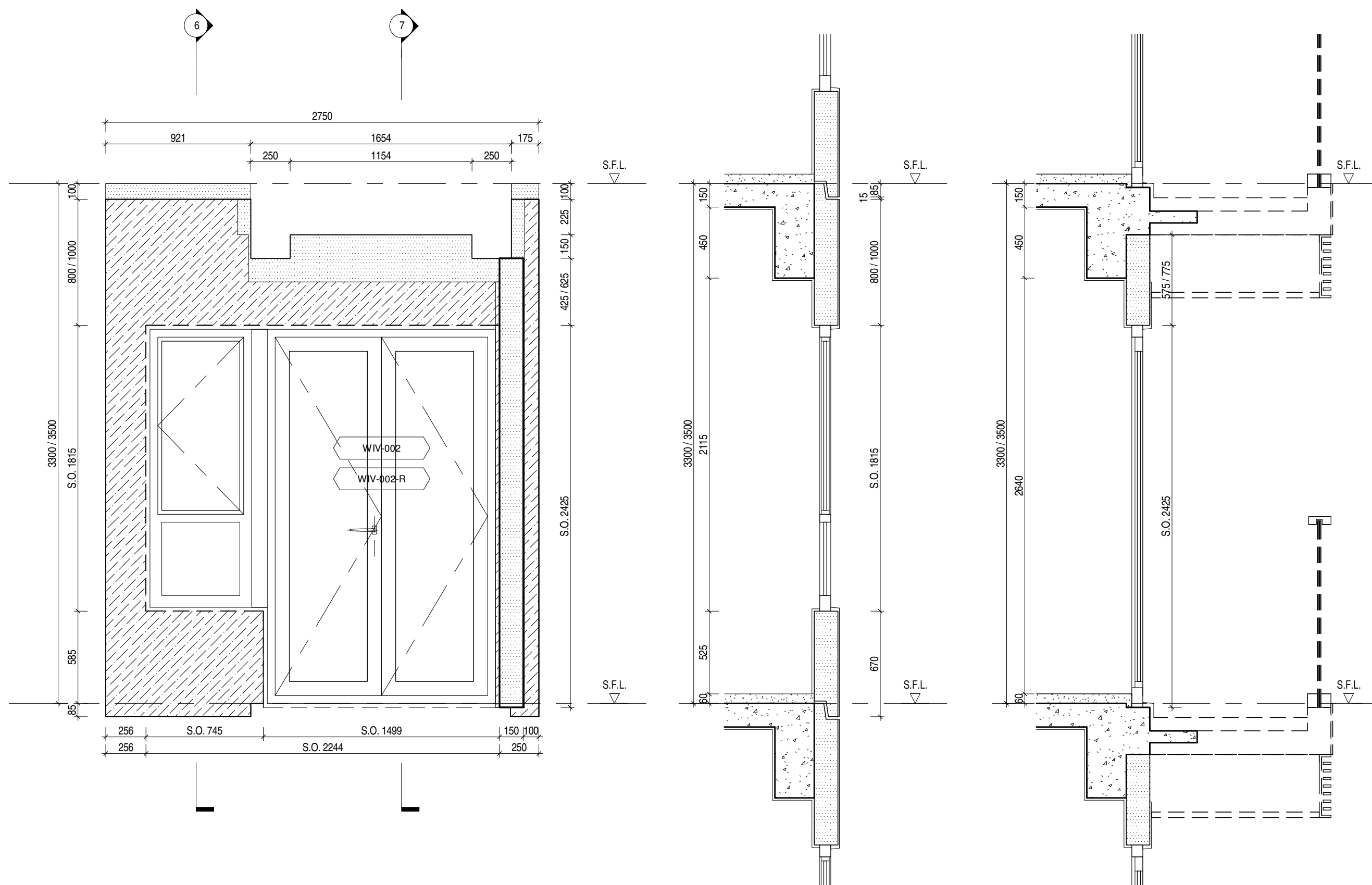
ELEVATION 5 1:25
