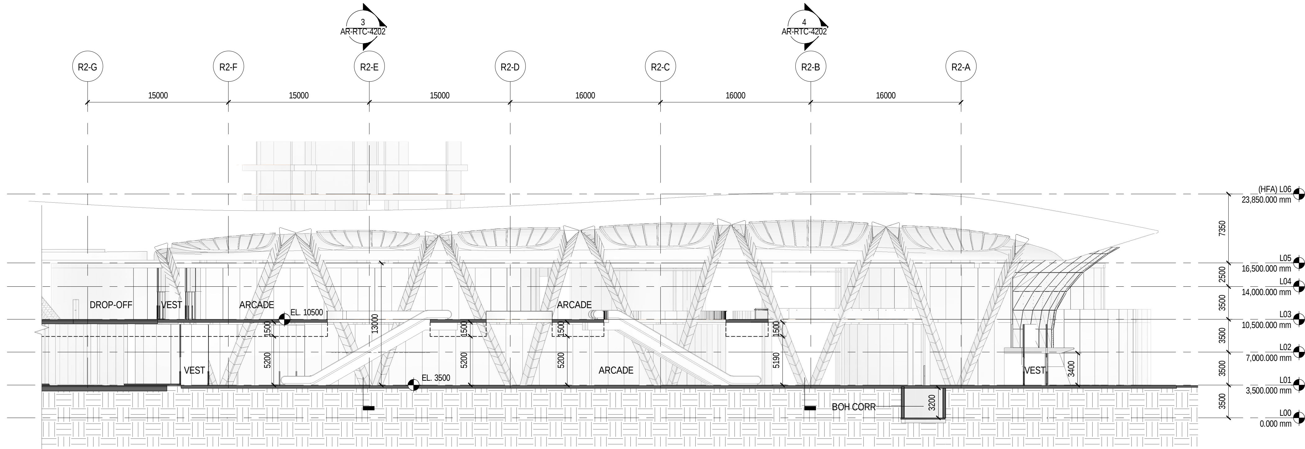
1 SECTION - INSPRIE SPACE SCALE: 1 : 250
