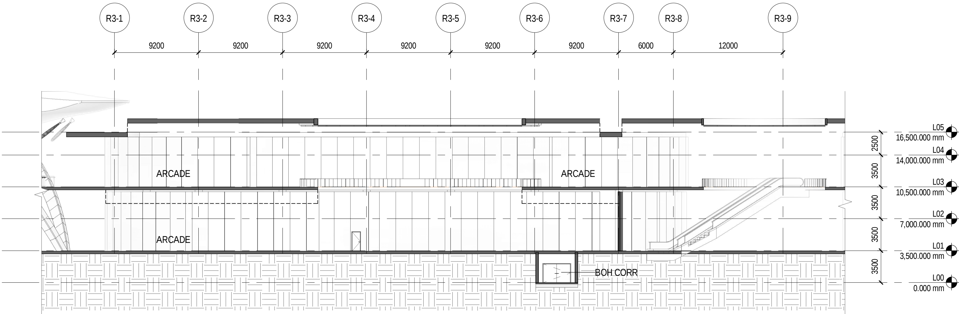
1 SECTION B SCALE: 1 : 250
