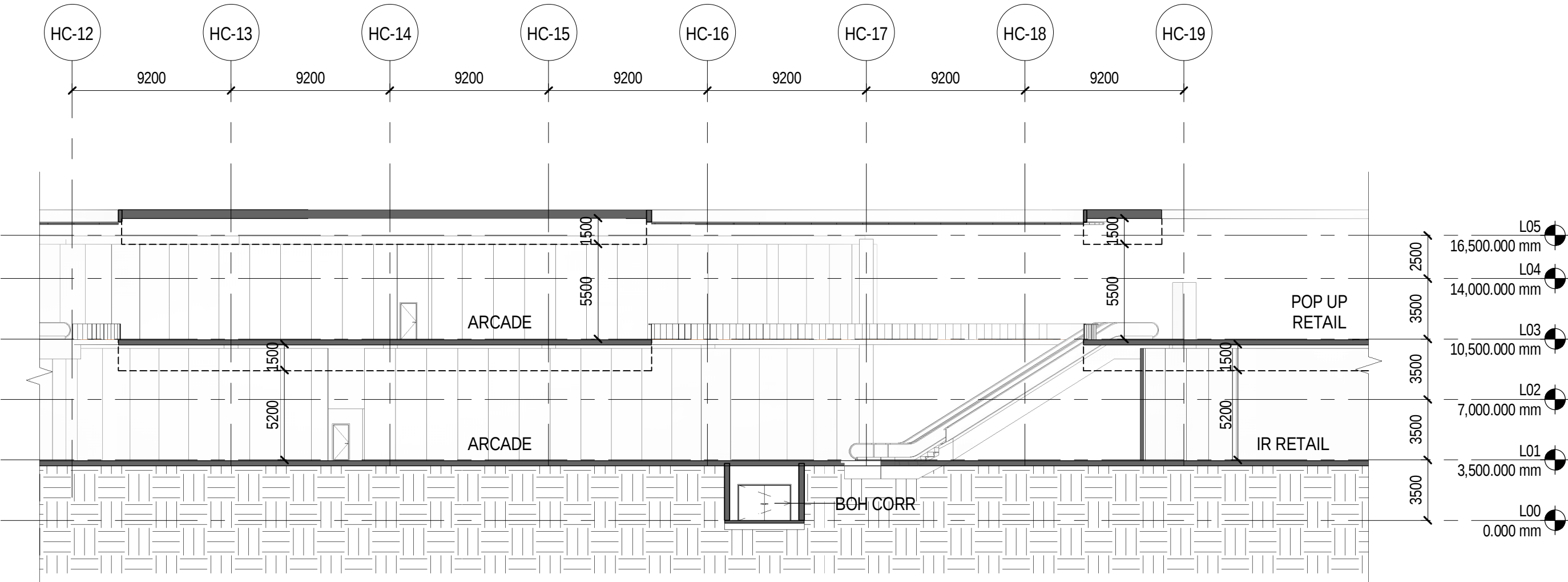
2 SECTION C SCALE: 1 : 250
