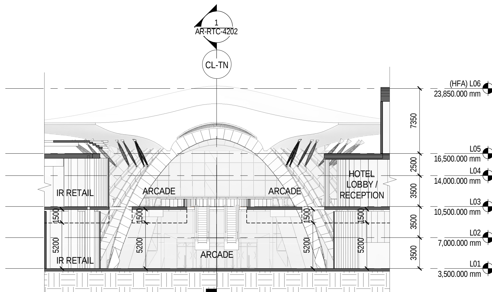
3 SECTION - INSPIRE SPACE - 3 SCALE: 1 : 250
