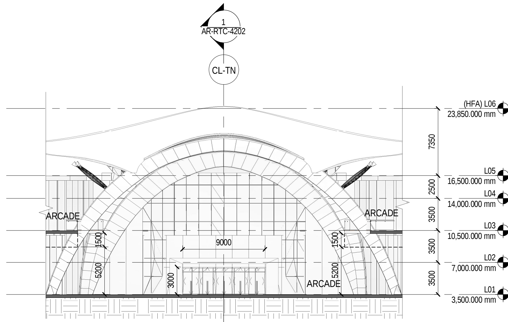
4 SECTION - INSPIRE SPACE - 4 SCALE: 1 : 250
