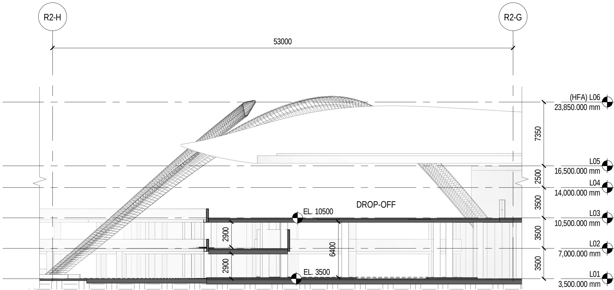
2 SECTION - INSPIRE SPACE - 2 SCALE: 1 : 250
