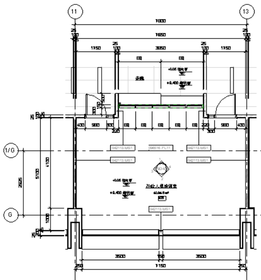
1 行政人员培训室平面图(高楼三层)1 1:50
