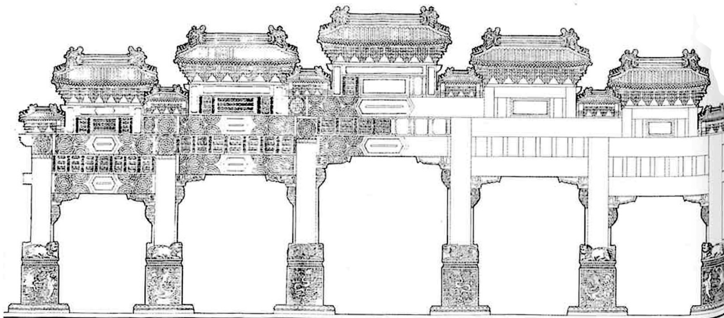
孝陵石牌坊正立面，钢笔墨线，1990
