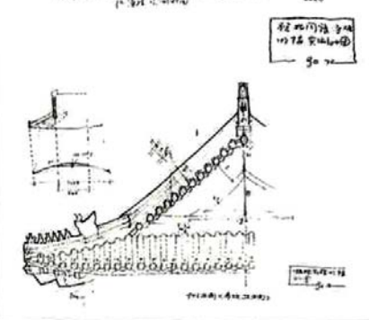
裕陵妃园寝测稿，铅笔草图，1990
