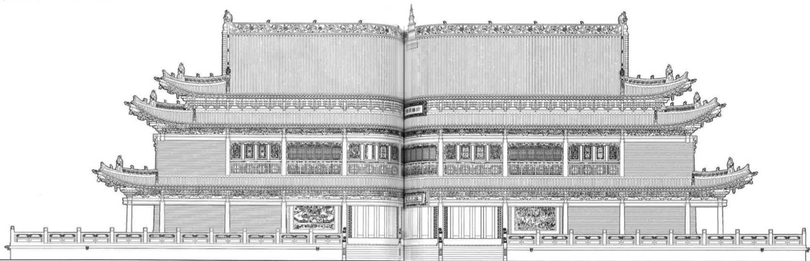
大佛寺大佛殿正立面图，计算机绘图，2000
