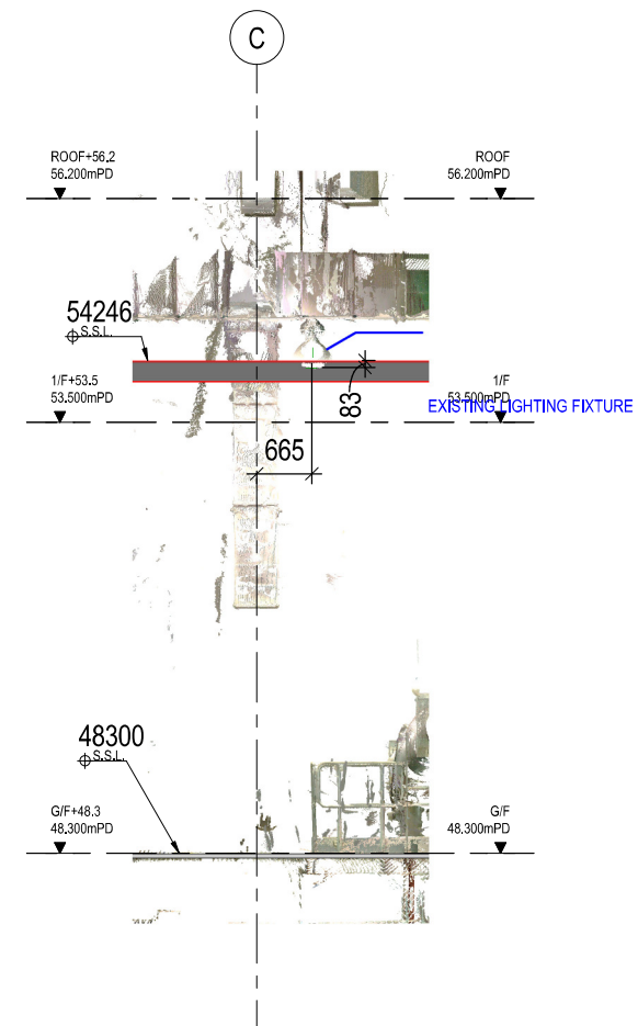
1 Section 1 - Callout 2 1 : 50
