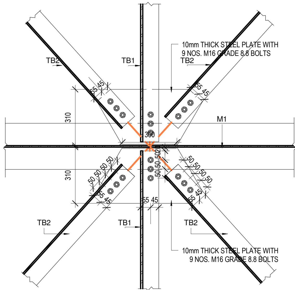
D1 SEC. D1 - D1 1 : 10
