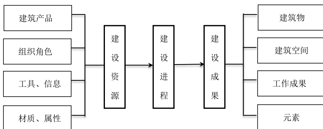
图 3.1.1 建筑信息模型分类结构
